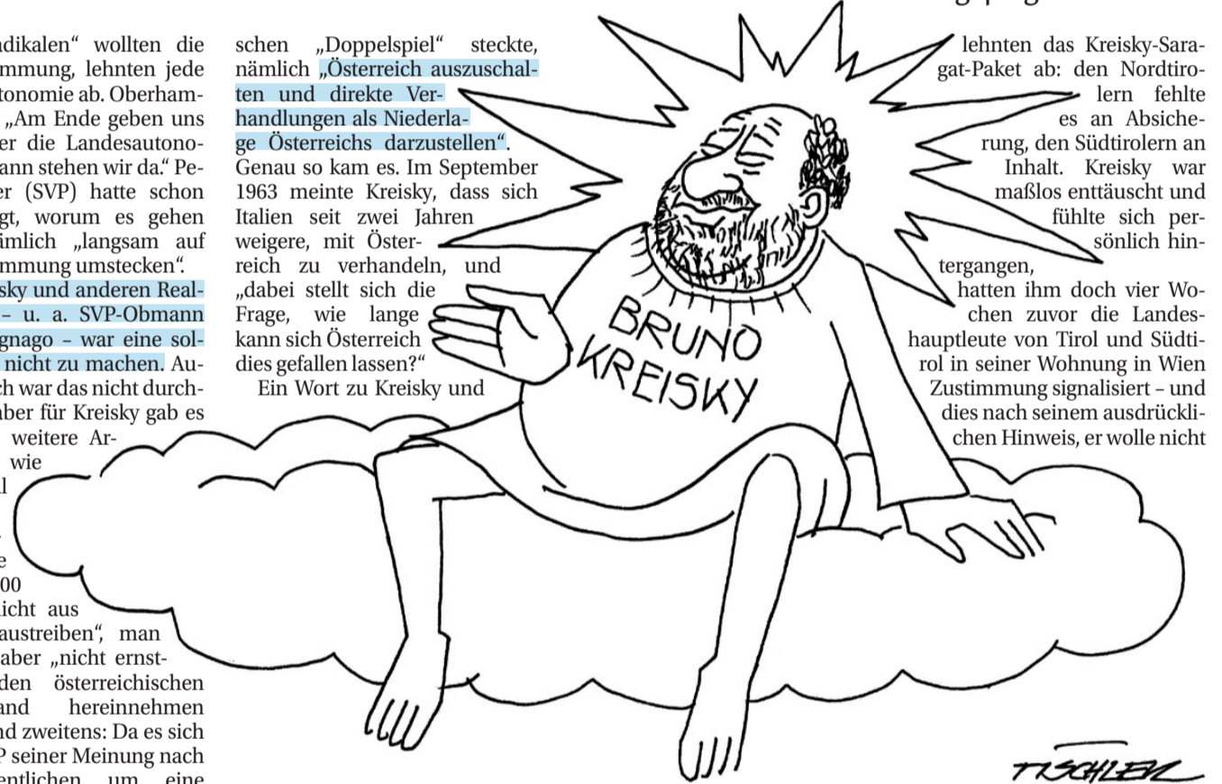
ÜBERSTRALENDER STERN
